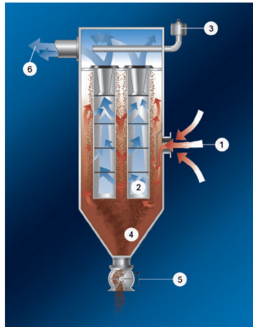
Принцип работы фильтра Deichmann
