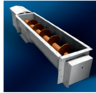
Лотковый шнековый транспортер
