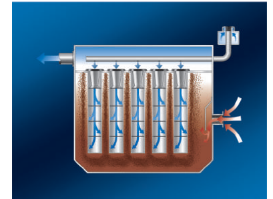
Очистка импульсом сжатого воздуха
