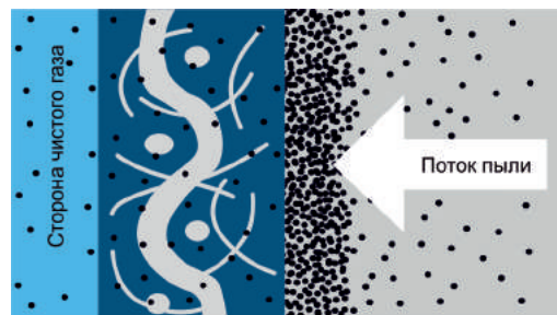
Принцип глубокой фильтрации*
