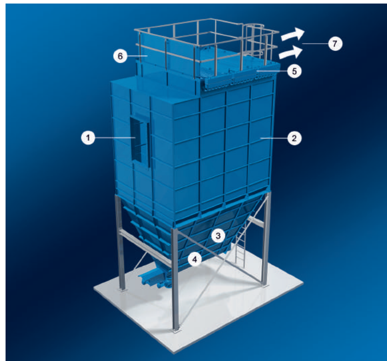
Установка рукавного фильтра Deichmann
