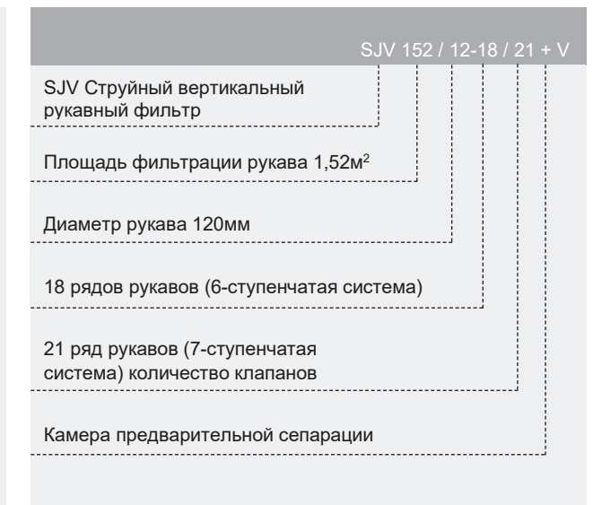
Общая площадь фильтрации 1,52м 2 x 18 x 21 = 575м 2
